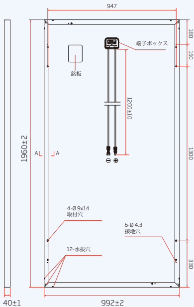
背面図
